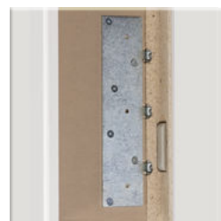
verstärktes Schließblech m. Stahlhalteplatte Nr. 35 Ansicht Futterrückseite
