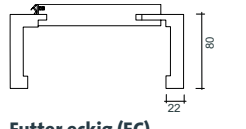
Futter eckig (EC), Bekleidungsbreite 80 mm
