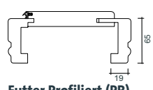
Futter Profiliert (PR), Bekleidungsbreite 65 mm
