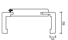
Futter Rundform (RF), Bekleidungsbreite 60 mm
