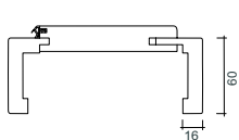
Futter Kleine Rundkante (KR), Bekleidungsbreite 60 mm
