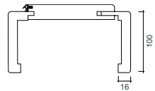
Futter Rundform (RF), Bekleidungsbreite 100 mm
