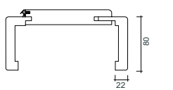
Futter Rundform (RF), Bekleidungsbreite 80 mm
