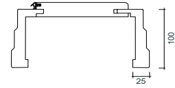
Futter Primo (PM), Bekleidungsbreite 100 mm
